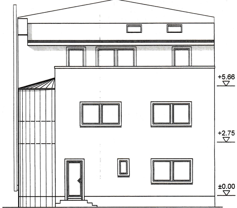
Ostansicht
